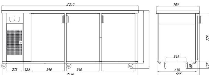
Габаритные размеры RT-3
