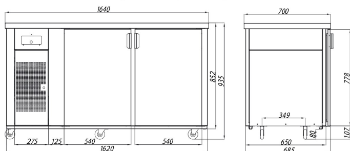
Габаритные размеры RT-2
