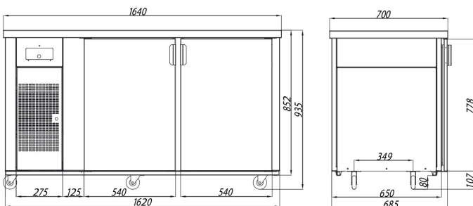
Габаритные размеры ВК-3
